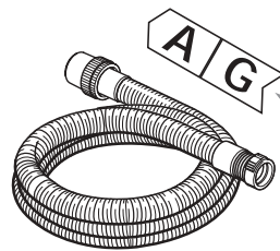
Saugschlauch Ø 36 mm Universal, 3 m mit Quicksystem Nr. 46948
